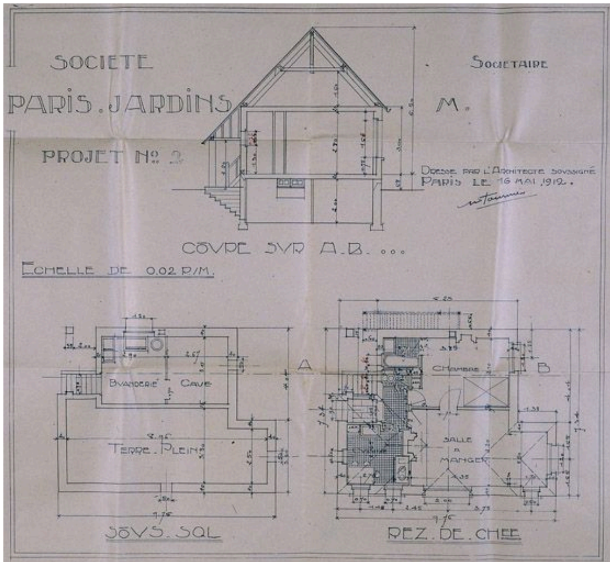
Plans du sous-sol et du rez-de-chaussée, coupe (projet n°2). (Société coopérative "Paris-Jardins" de Draveil, dossier 138)
