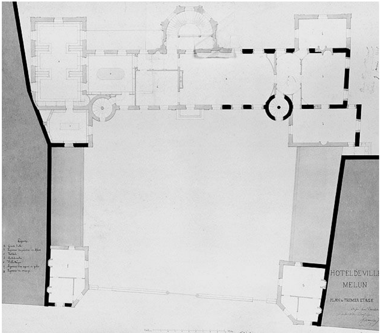
Album de 11 planches : projet d'hôtel de ville. Planche 7 : plan du premier étage. Papier aquarellé, 1844. (BM Melun. JJ 9)
