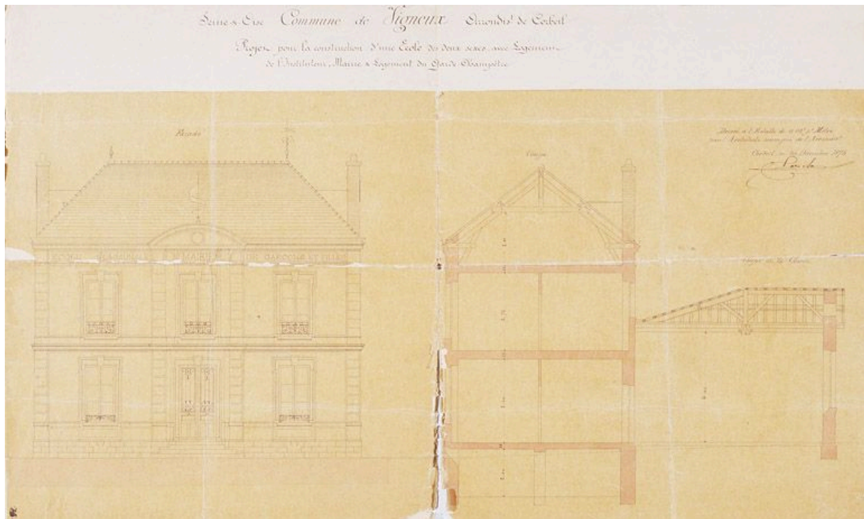
Projet de construction d'une école avec logement de l'instituteur, mairie et logement du garde-champêtre : façade principale et coupe. (AM Vigneux-sur-Seine, 1 M 2)
