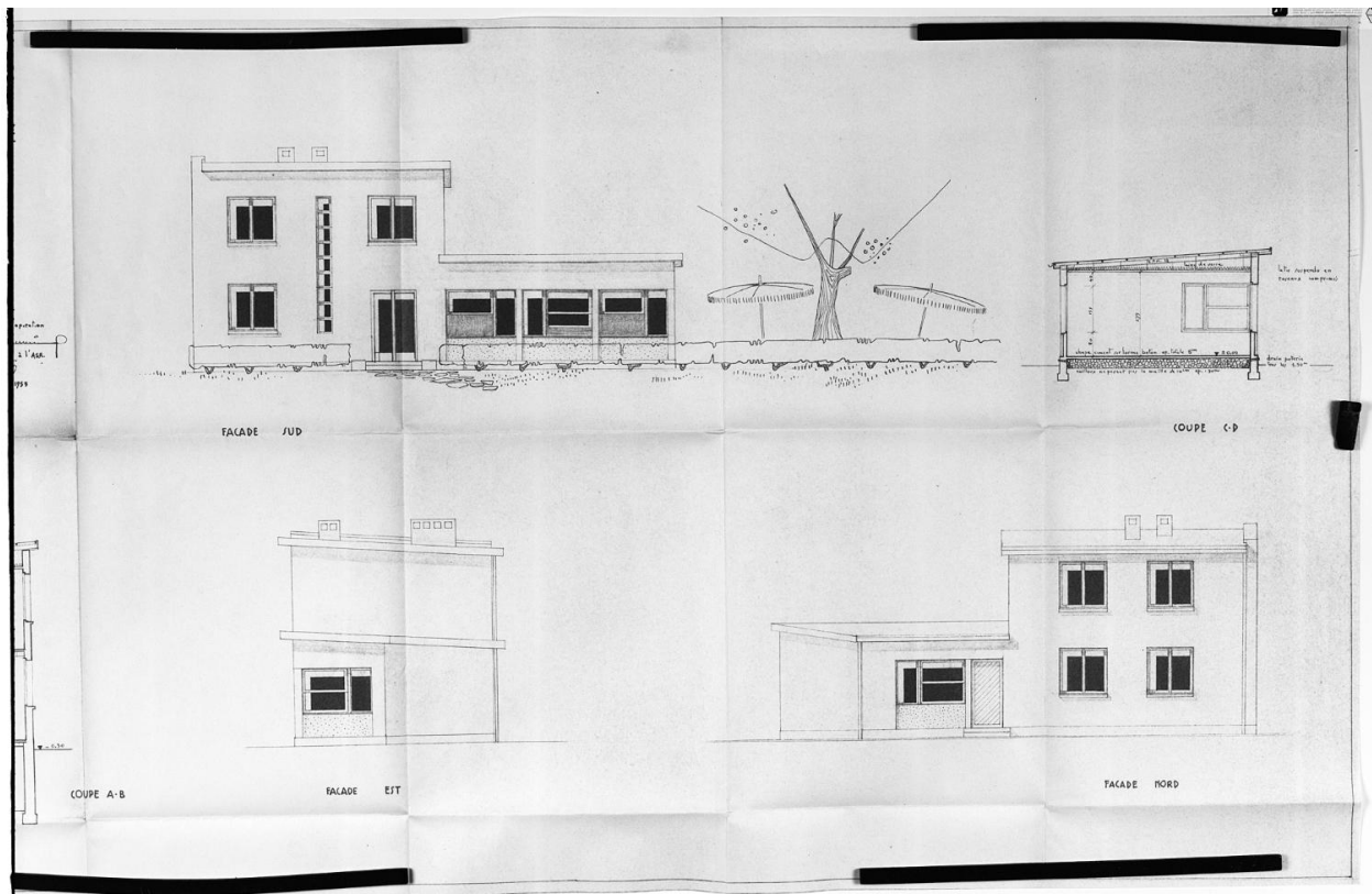
Elévations du pavillon reconstruit pour M. Rougery ; 31 décembre 1953, rectifié le 19 octobre 1954.
