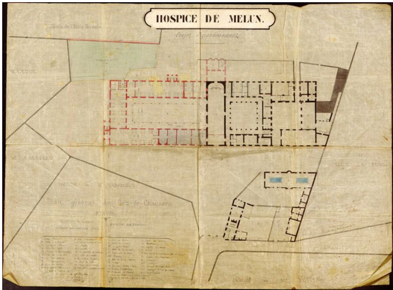
Hospice de Melun, projet d'agrandissement : plan général du rez-de-chaussée. Toile, 1861 (14 septembre). (AM Melun. 1 Fi 1039)
