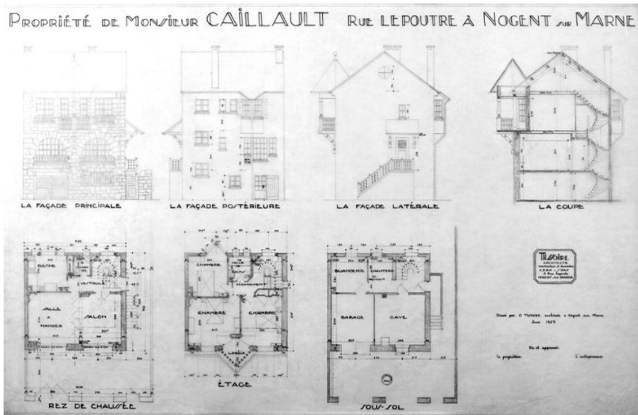
Plans du sous-sol, rez-de-chaussée et du premier étage; coupe et élévations antérieure, postérieure et latérale. Calque, 1929. (AD Val-de-Marne. 27 J 164)
