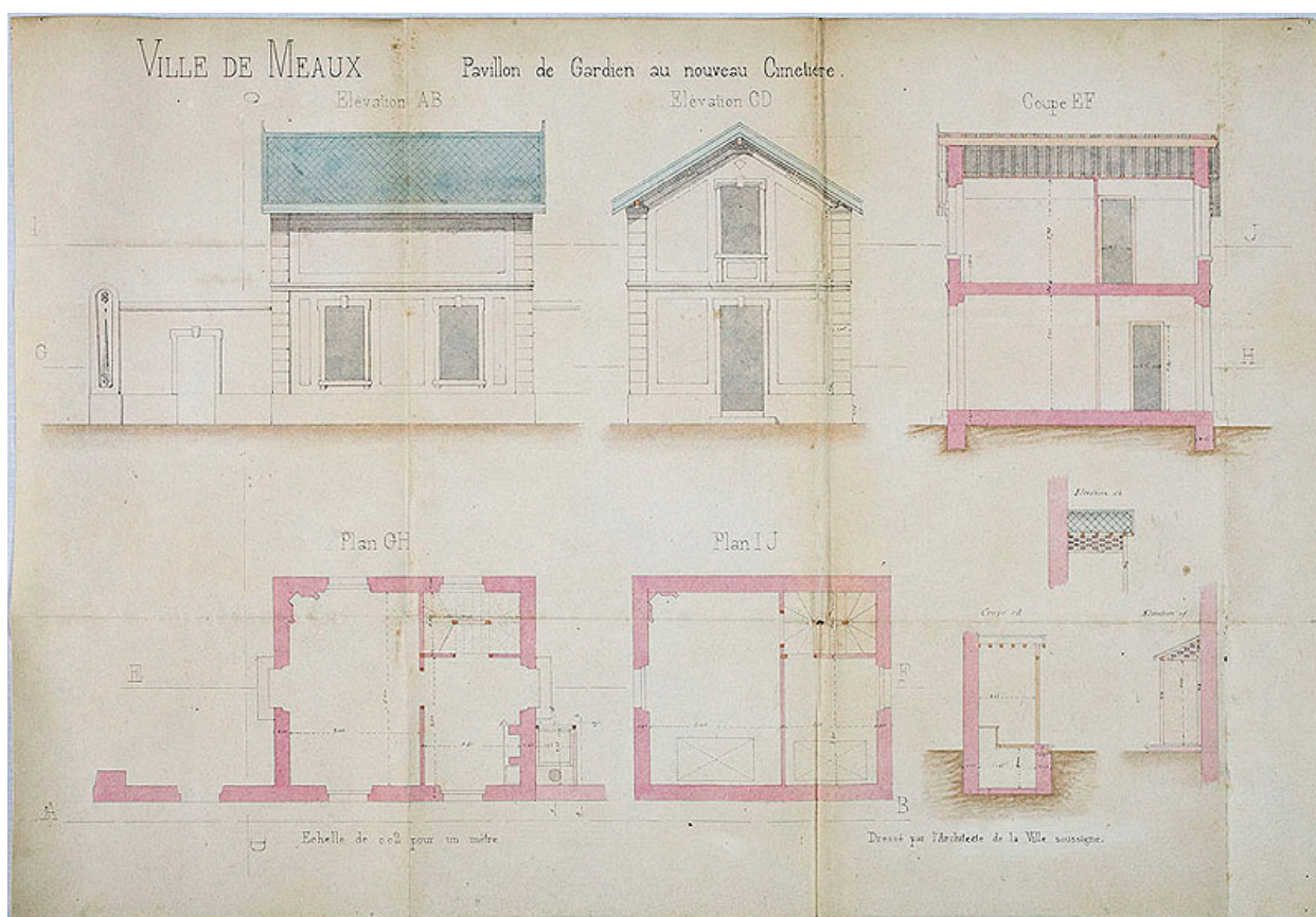
Pavillon de gardien au nouveau cimetière (2 élévations, 1 coupe, 3 plans) [1884]. Papier aquarellé. (AD Seine-et-Marne. 4 Op 284/13)
