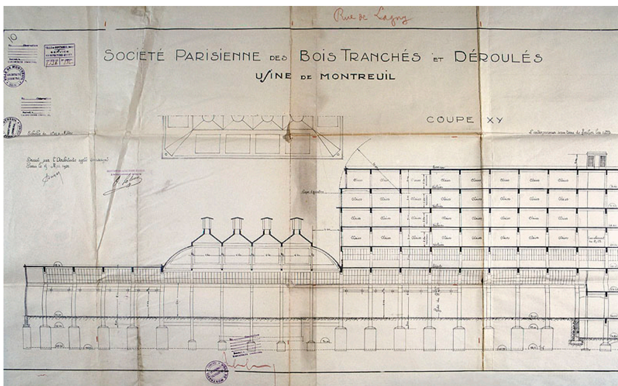
Coupe longitudinale, 1927, archives municipales de Montreuil.
