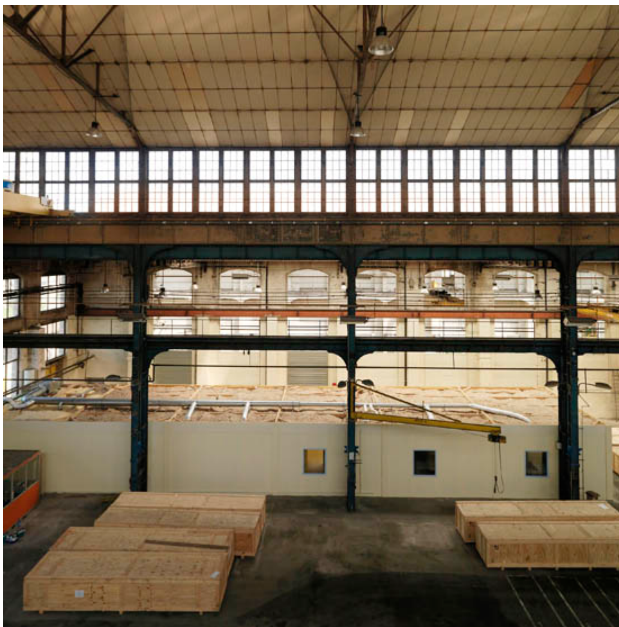
Vue intérieure de la nef centrale. Montage, machines-outils (1901-1903). Actuellement entreprise Jeumont Electric. Poteaux et charpente métallique.
