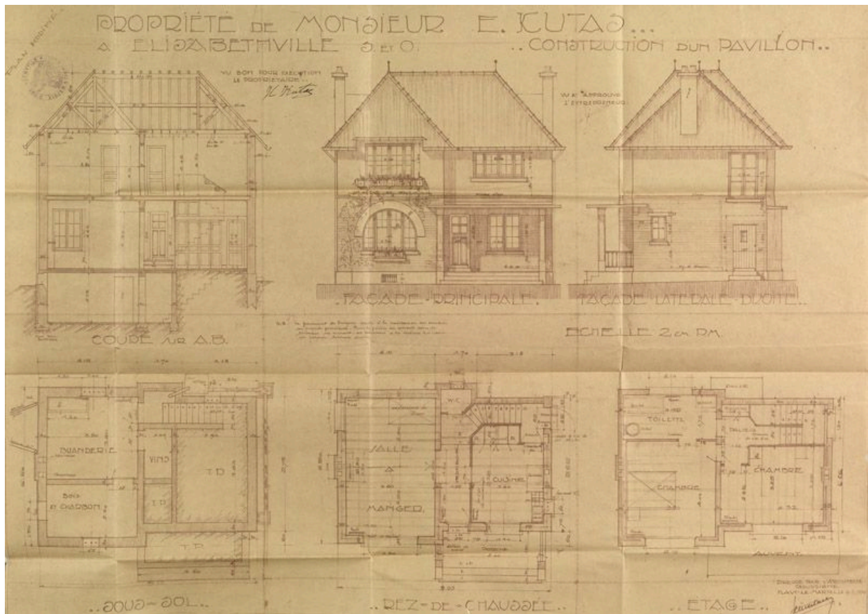
Plans de la maison de Monsieur E. Kutaz. Architecte : A. Schiketans, 1932 (AM Aubergenville).
