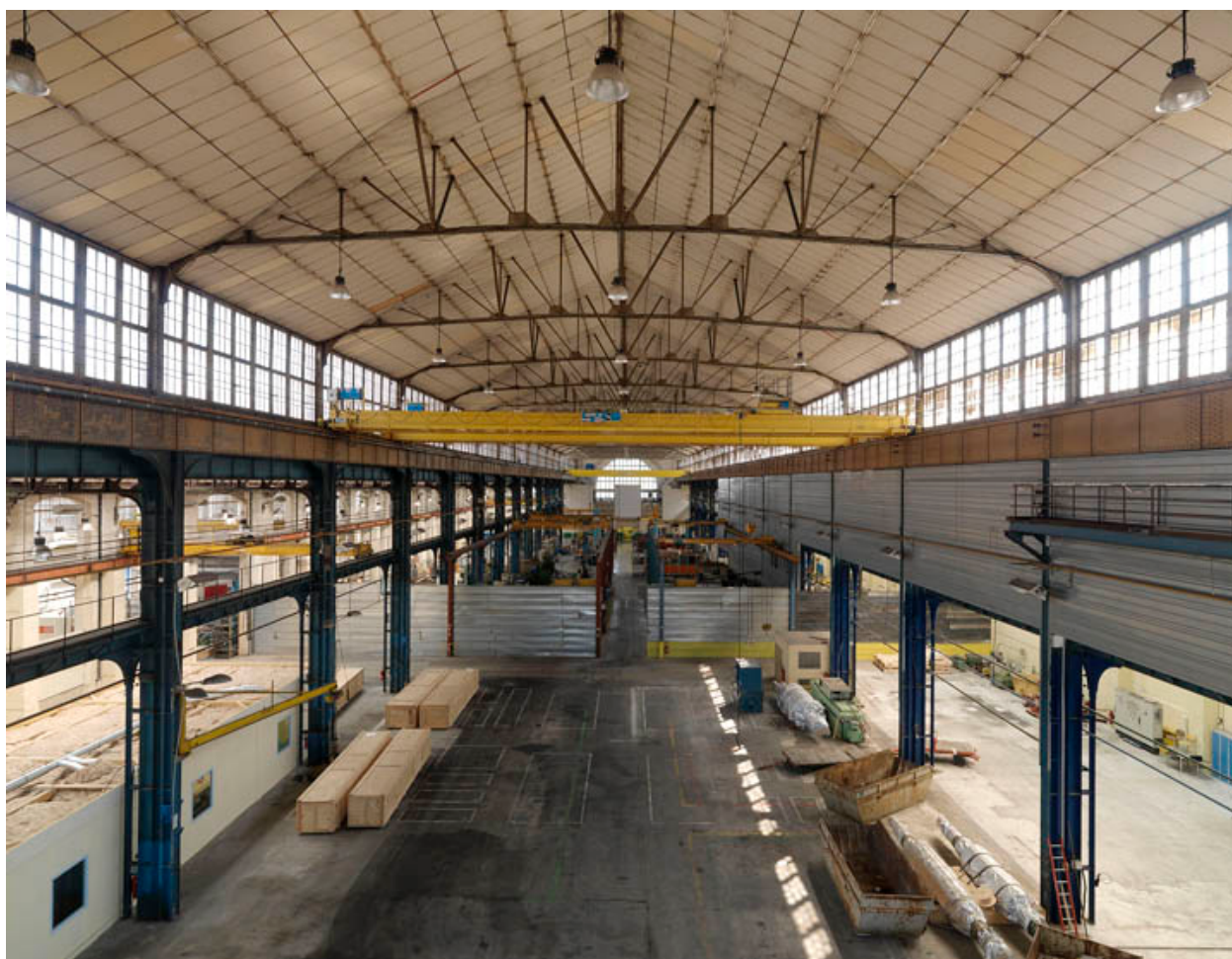
Vue intérieure de la nef centrale. Montage, machines-outils (1901-1903). Actuellement entreprise Jeumont Electric. Poteaux et charpente métallique.
