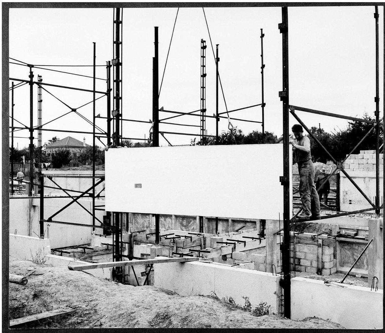
Installation d'éléments préfabriqués sur armature de métal, 1959.
