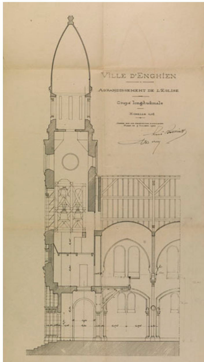
Coupe longitudinale de l'agrandissement au niveau du clocher et des nouvelles travées construits en 1926. (AM Enghien-les-Bains, M48)
