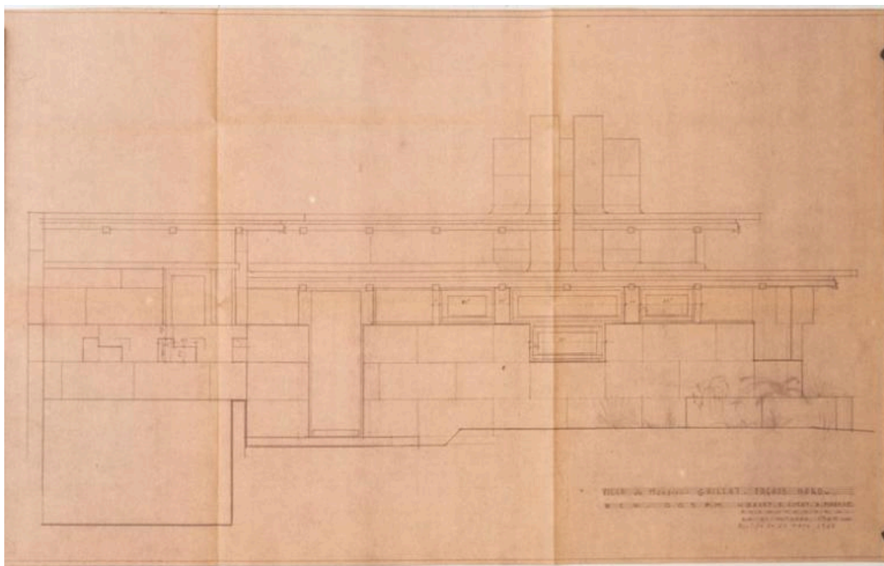
Façade Nord (extrait du permis de construire).
