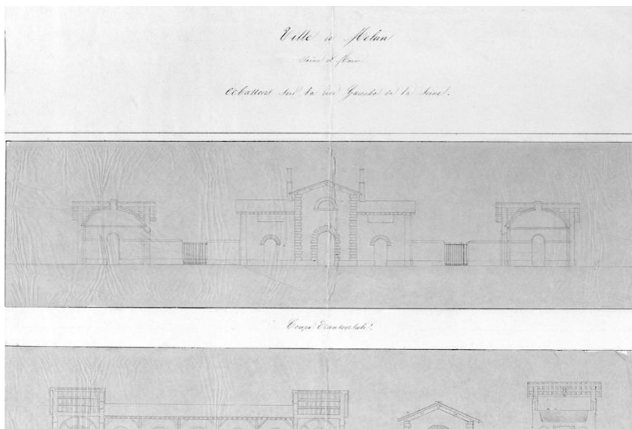
Ville de Melun, abattoirs sur la rive gauche de la Seine : coupe transversale. Encre sur calque, 30 décembre 1839. (AM Melun. 1 Fi 384)
