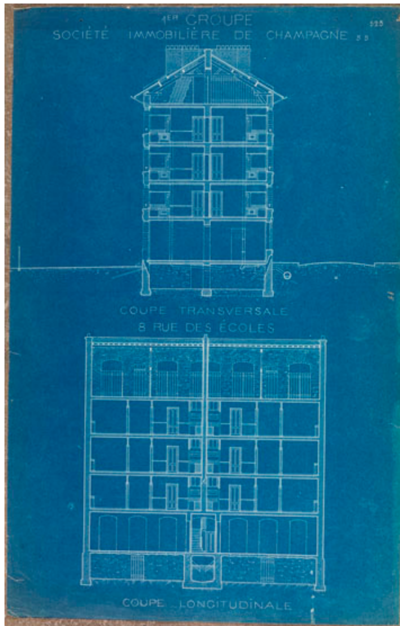
Plan. Société immobilière de Champagne. Coupes transversale et longitudinale..1er groupe, 8 rue des écoles.
