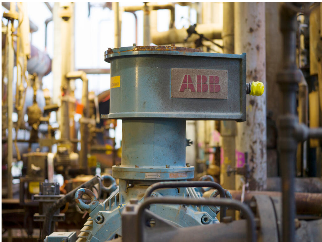
Unités Ouest - Zone de distillation (Unité 612). Branchement électrique ABB d'un moteur de pompe.
