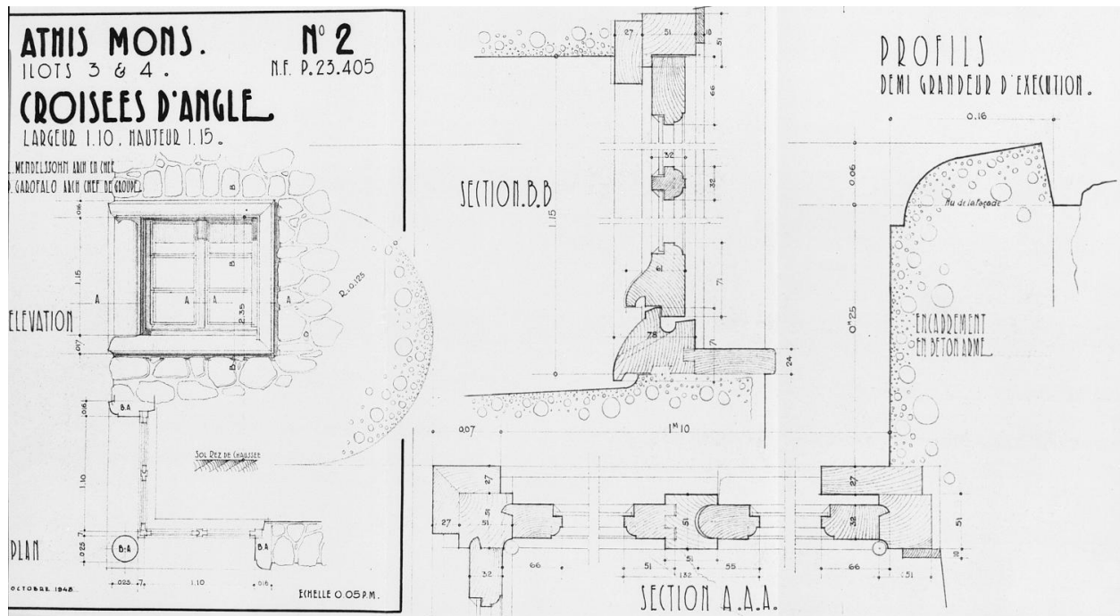
Ilots 3 et 4 : élévation et profil des croisées d'angle ; L. Mendelssohn architecte en chef, P. Garofalo architecte chef de groupe, octobre 1948.
