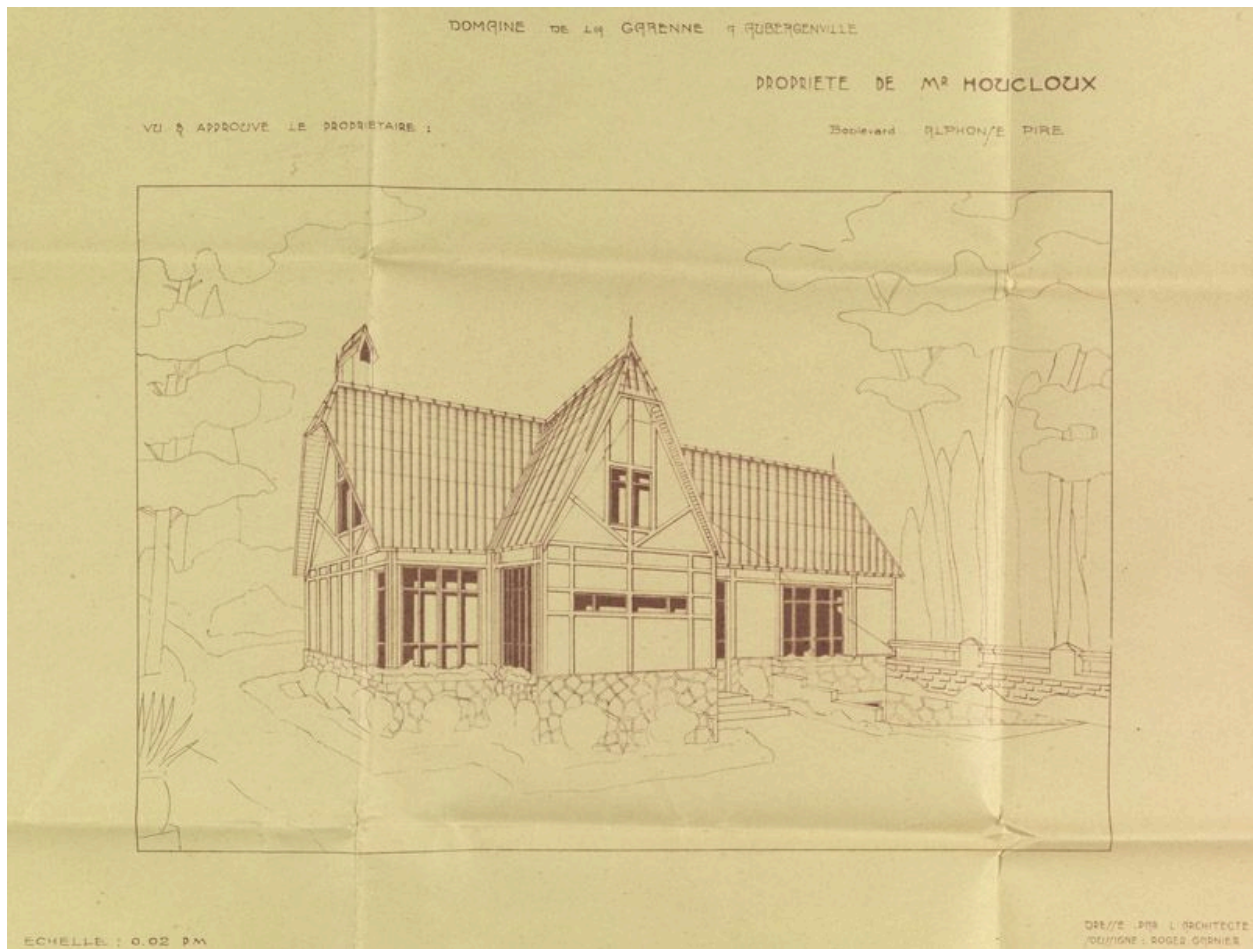
Elévation de la maison de M. Houcloux, boulevard Alphonse Pire. Architecte : Roger Garnier, 1933 (AM Aubergenville).
