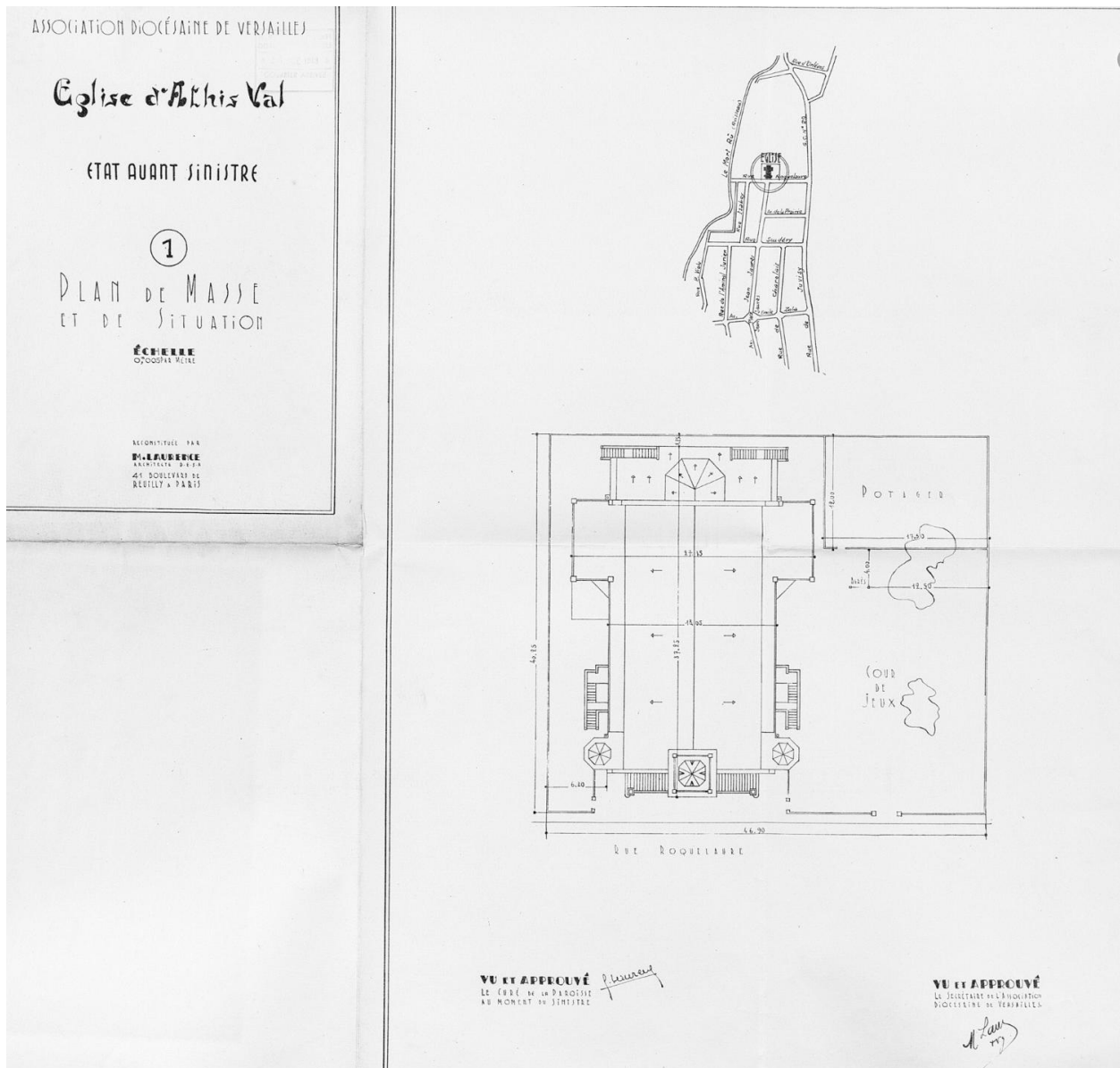
Plan de masse et de situation, reconstitué par Maurice Laurence, architecte, [1951].
