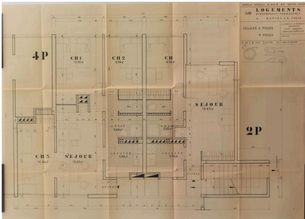
Plan détaillé des cellules de 2 pièces et 4 pièces des logements HLM de Candilis et Brunache. Mantes-la-Jolie. Permis de construire, 68/55.
