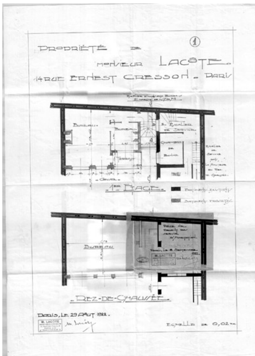
Rez de chaussée immeuble sur cour, propriété de Monsieur Lacôte. -Plan, 1922. (Archives de Paris, VO11 1131).
