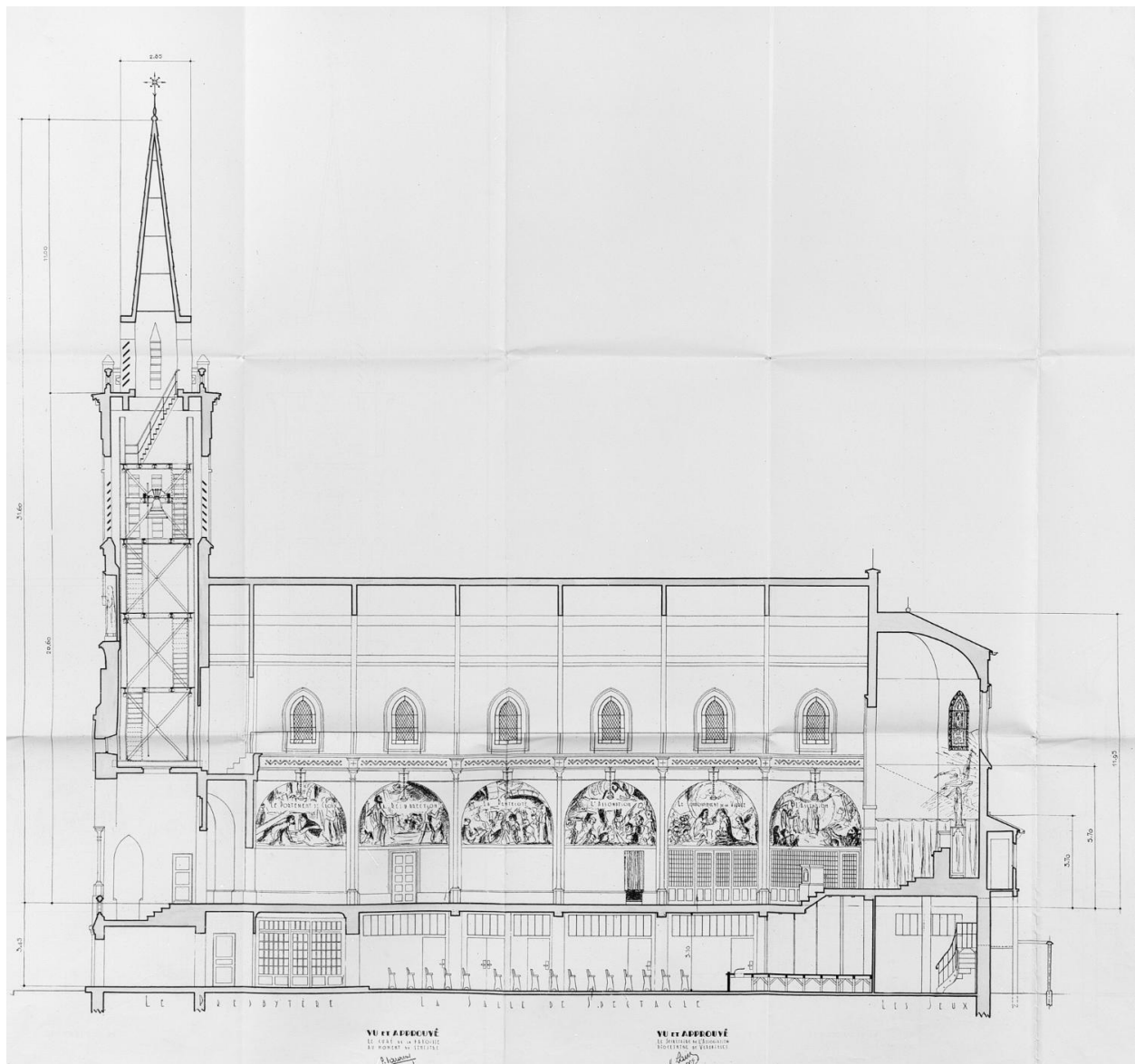
Coupe longitudinale reconstituée par Maurice Laurence, architecte. [1951].
