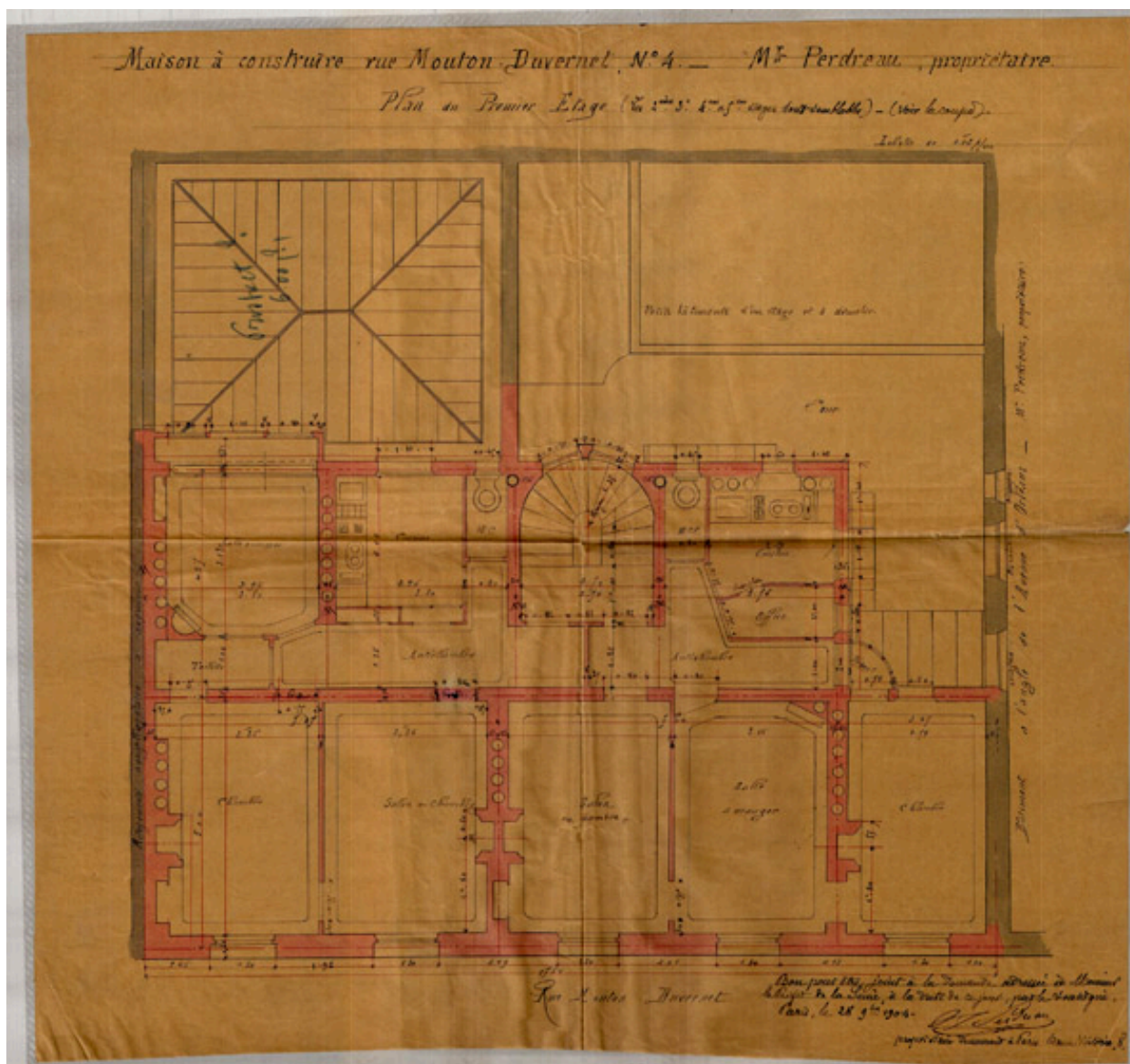
Plan du premier étage et des étages suivants d'une maison à construire au 4 de la rue. 1904. (Archives de Paris VO11 2306)
