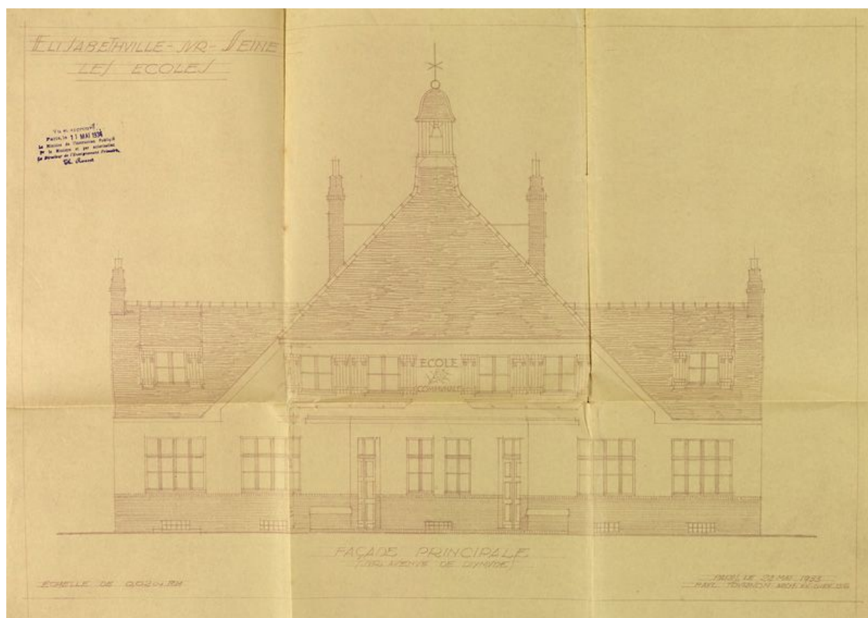
Elévation de la façade principale de l'école de la Reine Astrid construite en 1931. Tirage, 1930. (AM Aubergenville).
