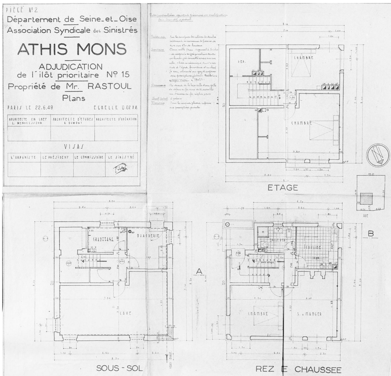
Plans (sous-sol, rez-de-chaussée et étage) de la maison reconstruite dans l'îlot 15 pour M. Rastoul (20, rue du Vercors) ; architecte en chef Léo Mendelssohn, G. Dumont, architecte d'études, Faine architecte d'opération, 22 juin 1949.
