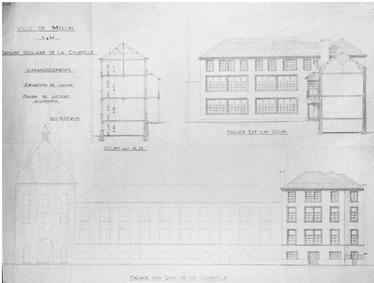
Groupe scolaire de la Courtille. Agrandissements : élévations et coupe..Papier, s.d. (AM Melun. 1 Fi 631)
