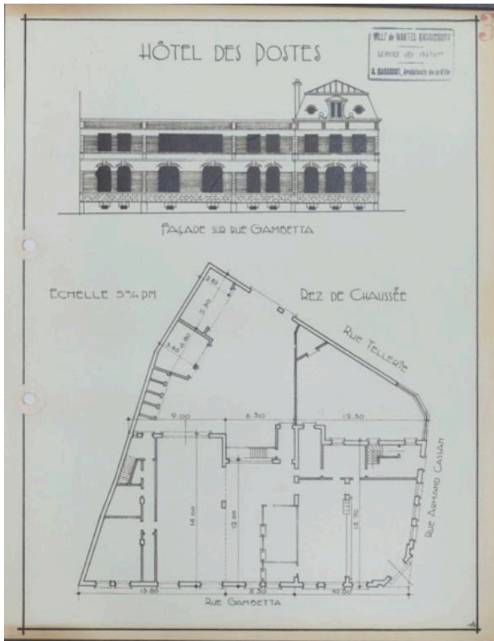
Elevation et plan vers 1940. (AM. Mantes-la-Jolie, 1 M 1)
