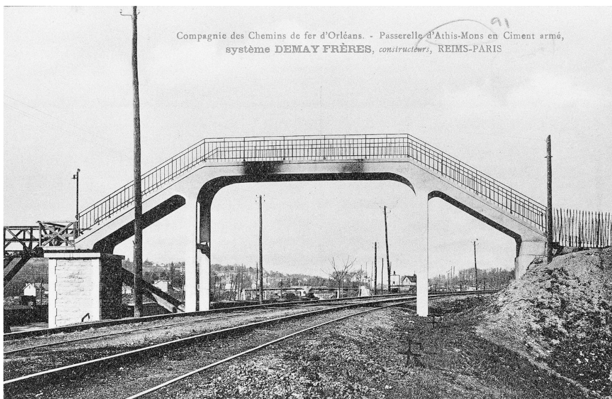
La passerelle en ciment armé dans le prolongement de la passerelle de l'avenue de Seine.
