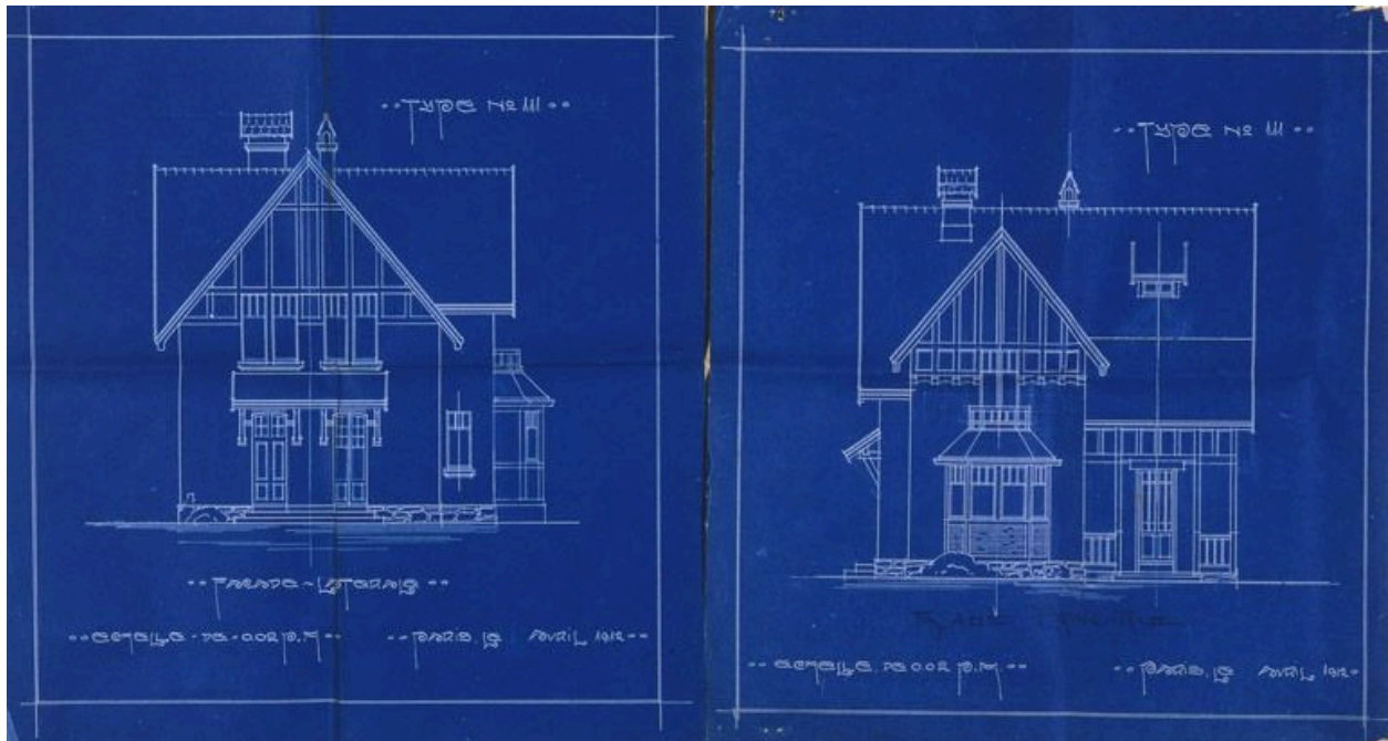
Plan d'un pavillon du type 111 : élévations. (Société coopérative "Paris-Jardins" de Draveil, dossier 179)
