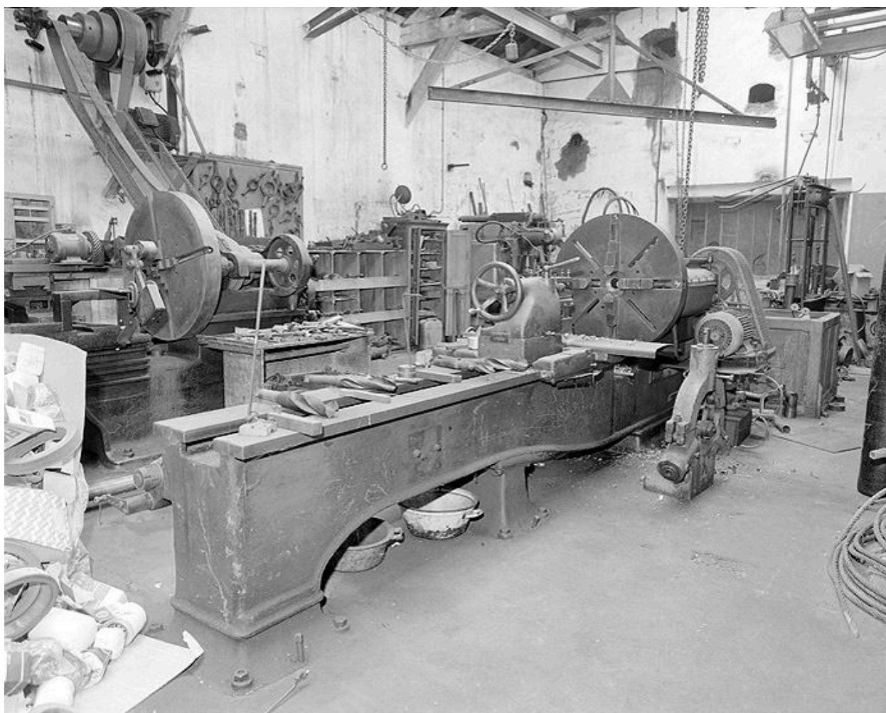
Petit tour pour fabrication des arbres d'hélices.
