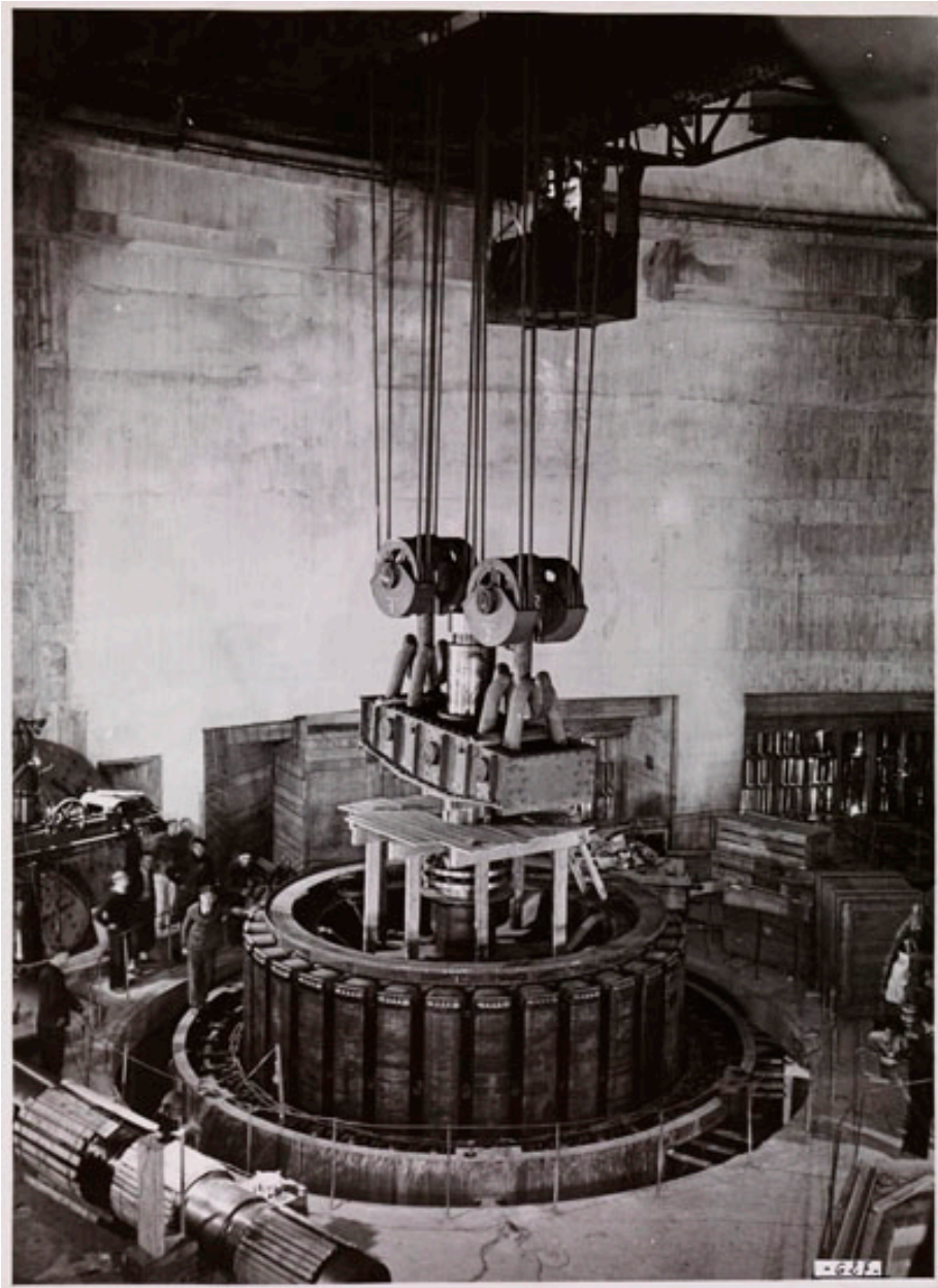
Photo ancienne. Présentation du rotor d'un alternateur.
