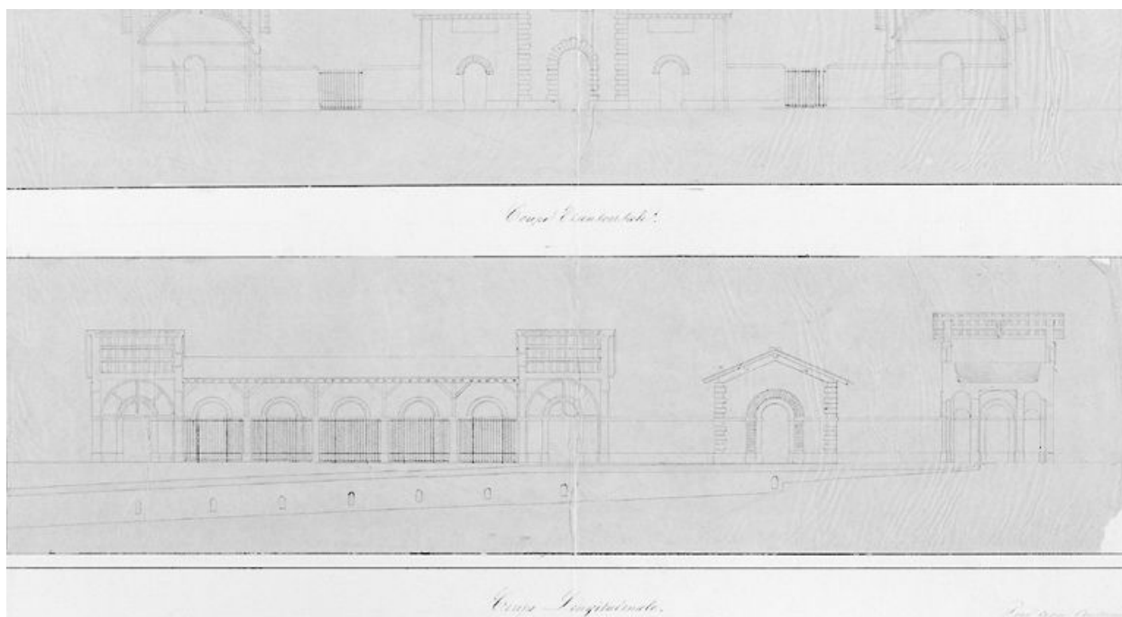
Ville de Melun, abattoirs sur la rive gauche de la Seine : coupe longitudinale. Encre sur calque, 30 décembre 1839. (AM Melun. 1 Fi 384)
