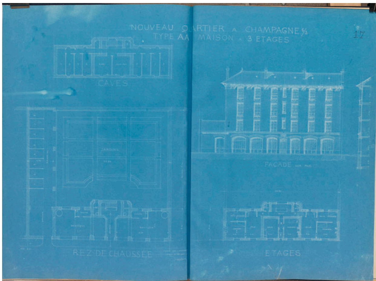
Plan. Edmond Delaire. Projet pour "le nouveau quartier" de Champagne-sur-Seine. Type AA maison à trois étages.
