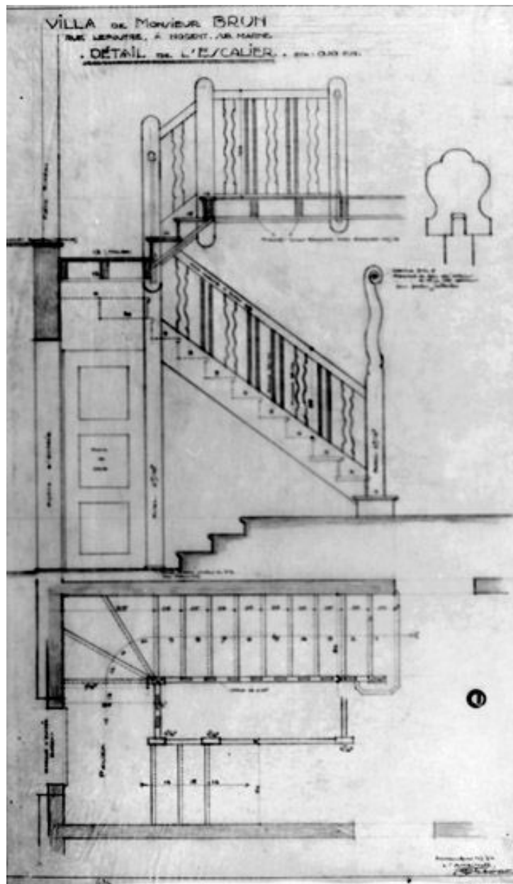
Plan et coupe de l'escalier. Calque, 1934. (AD Val-de-Marne. 27 J 163)
