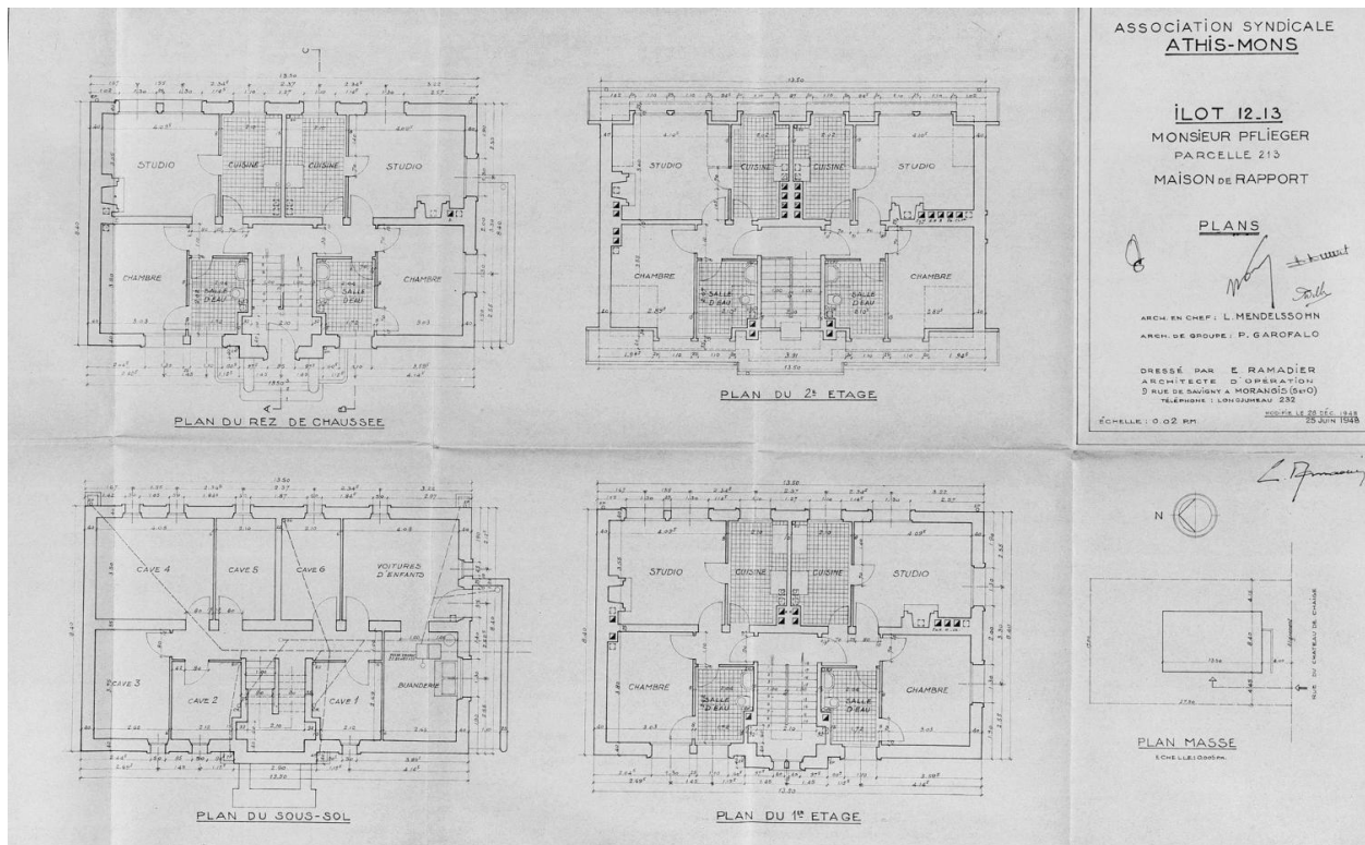
Plans de l'immeuble reconstruit pour M. Pflieger dans l'îlot 12-13, parcelle 213, par E. Ramadier, architecte d'opération, 25 juin 1948.
