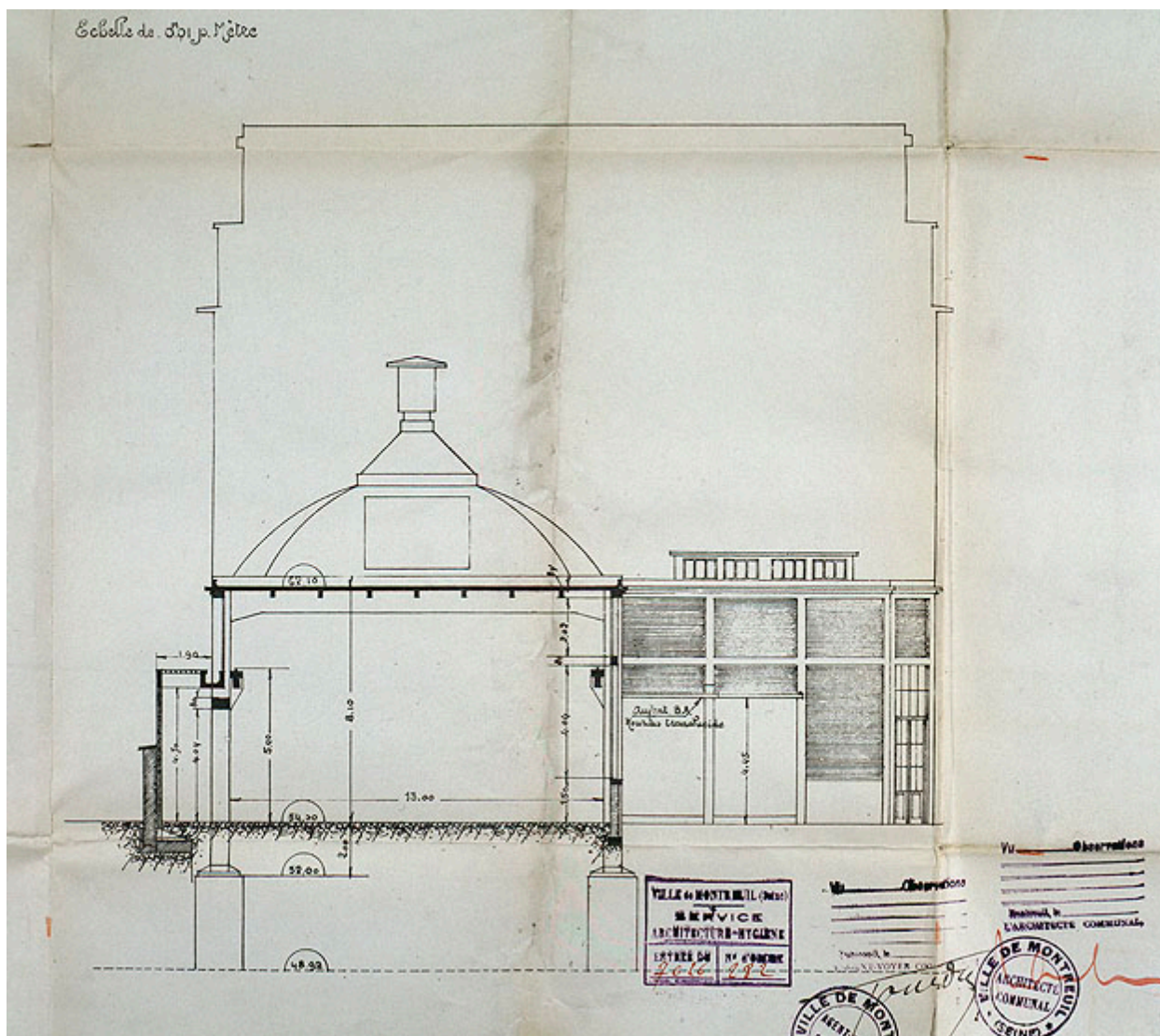
Coupe des étuves, 1927, archives municipales de Montreuil.
