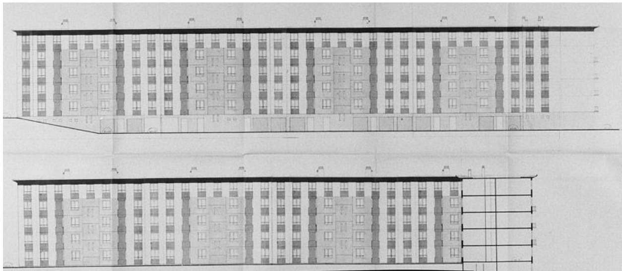
Bâtiment long R + 5 : plans des façades principales, dressés par J. L'Hernault, 16 juillet 1965. (AM Vigneux-sur-Seine, 80 W 29, dossiers 57-58)
