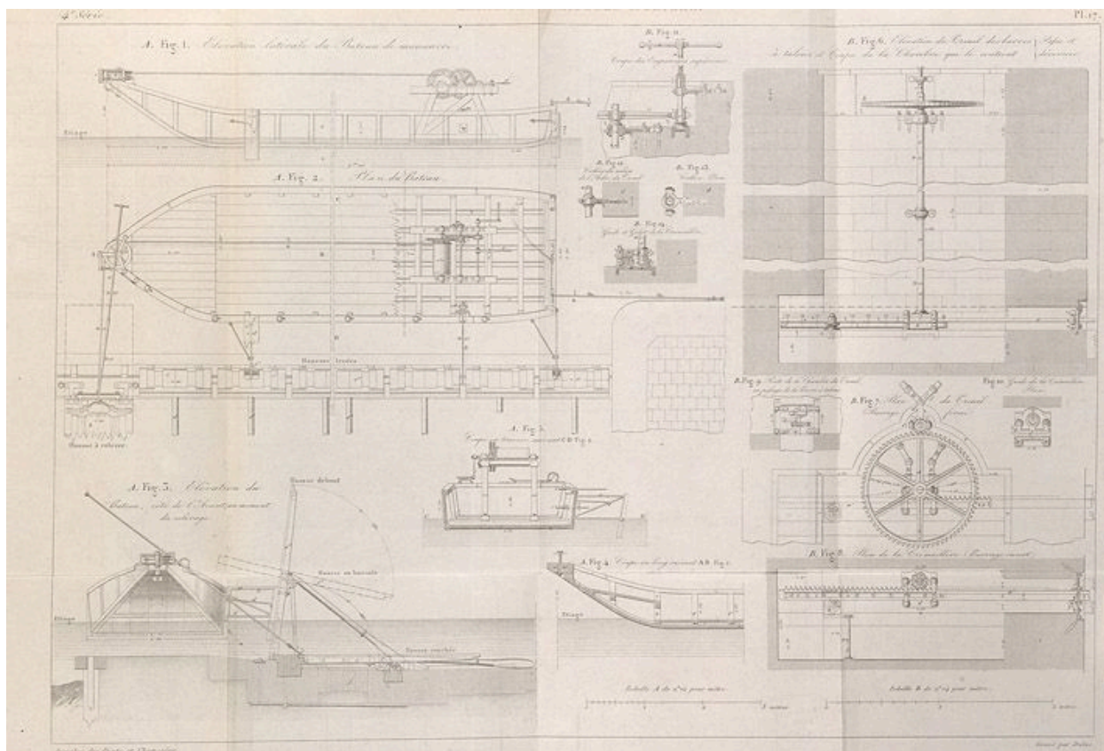
Barrages à hausses mobiles, bateau de manoeuvre. Tiré de : Mémoire sur les barrages à hausses mobiles / M. Chanoine et M. de Lagrené. In Annales des Ponts et Chaussées, 2e semestre, 1861, n° 21, pl. 15-17.
