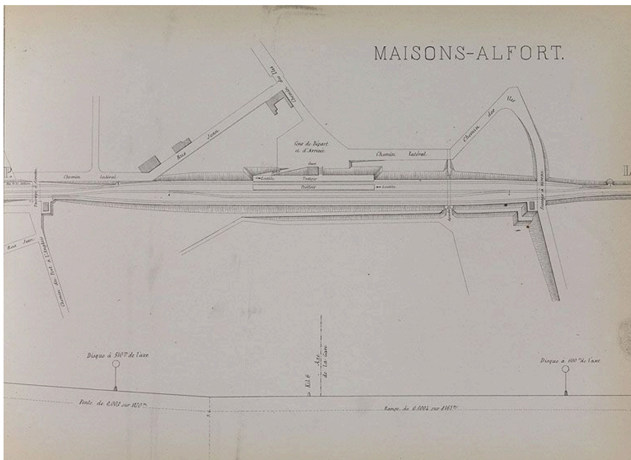
Chemin de fer de Paris à Lyon. Profil général de la ligne ; plans et profils détaillés des gares, s.d. [vers 1852-55], [d'après Lagrière, ancien chef de gare de Bercy]. Plan de la gare de Maisons-Alfort. (Ecole nationale des ponts et chaussées)
