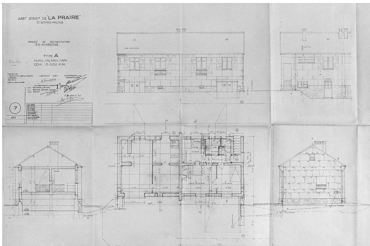
Plans, façades et coupe d'un pavillon du type A ; 24 juin 1948.
