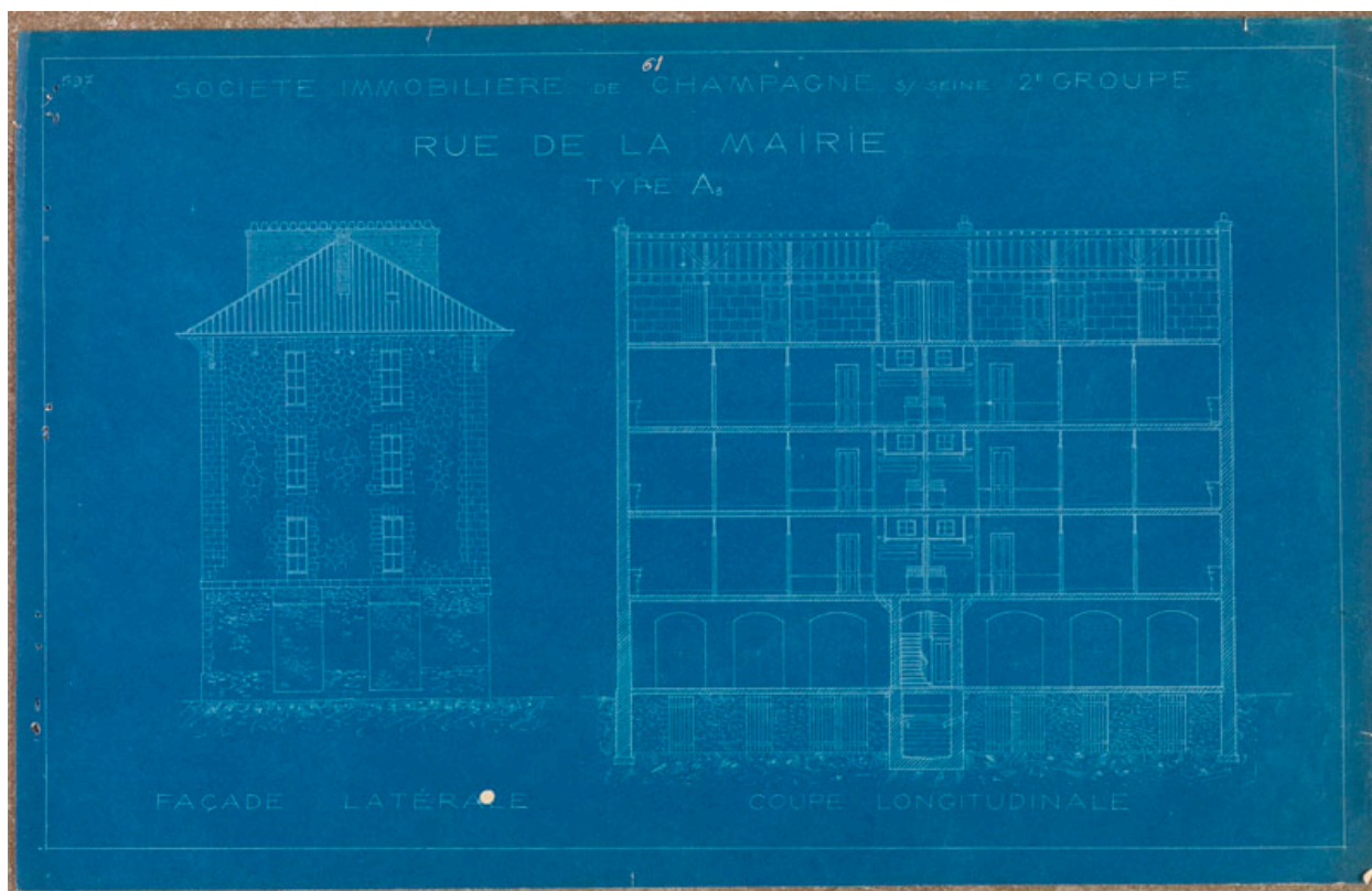
Plan. Société immobilière de Champagne. Façade et coupe longitudinale. 2e groupe type A rue de la mairie.
