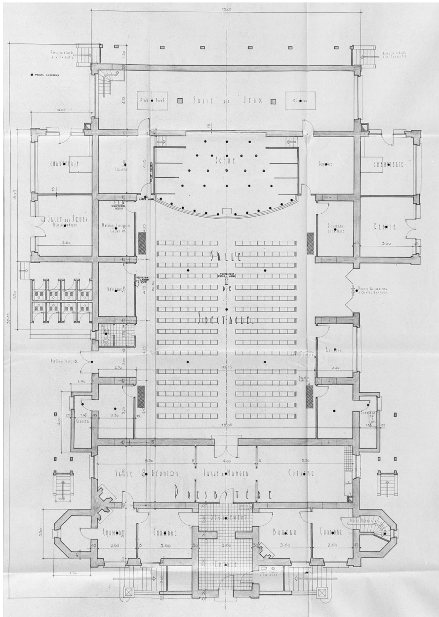
Plan du sous-sol (aménagé en salle de spectacle et locaux annexes), reconstitué par Maurice Laurence, architecte, [1951].
