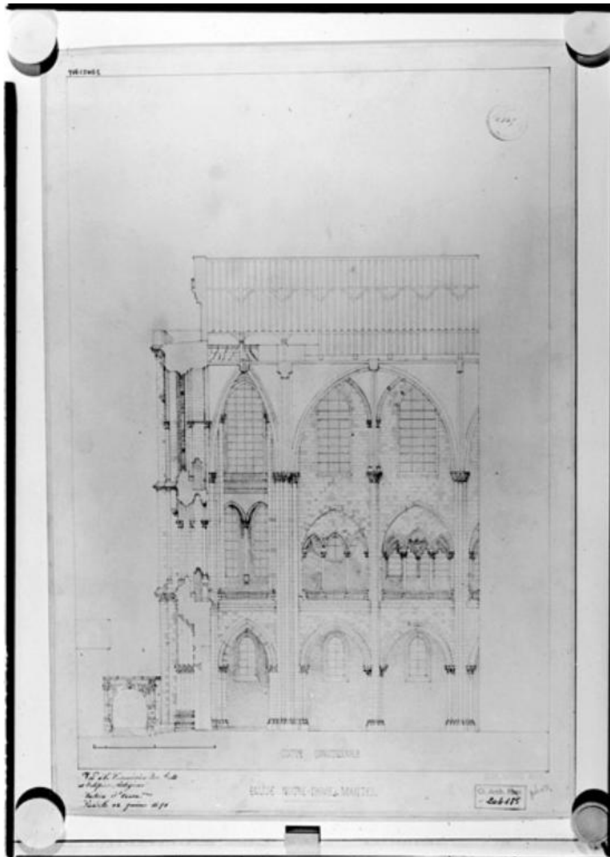
Relevé Monuments Historiques. A. Durand (1851). Coupe longitudinale.
