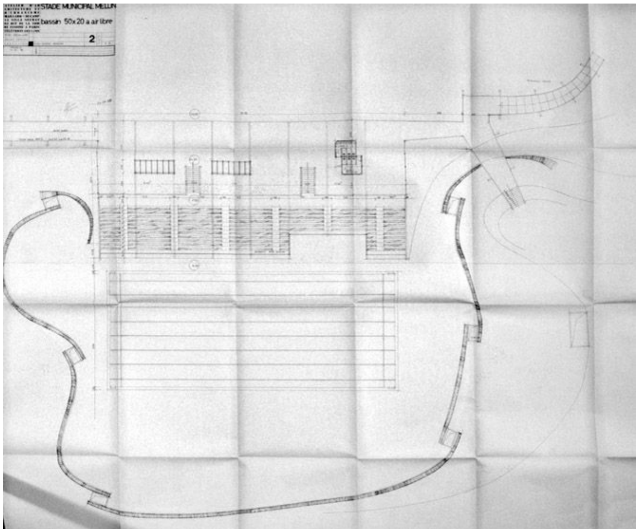
Bassin découvert : plan au niveau des gradins. Tirage d'architecte, 14 octobre 1966. (AM Melun. 466 W 84)
