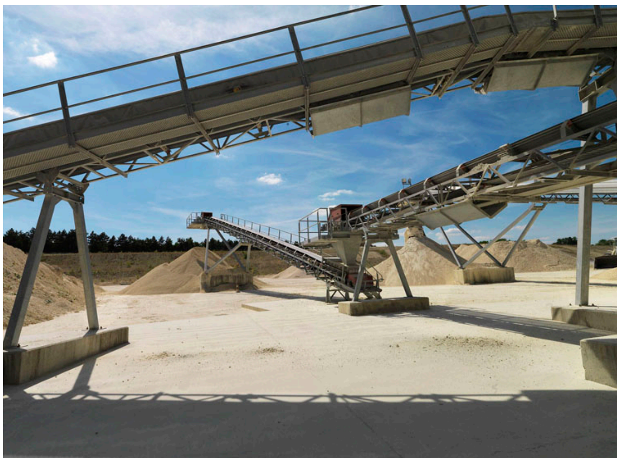
Plateforme - installation secondaire.
