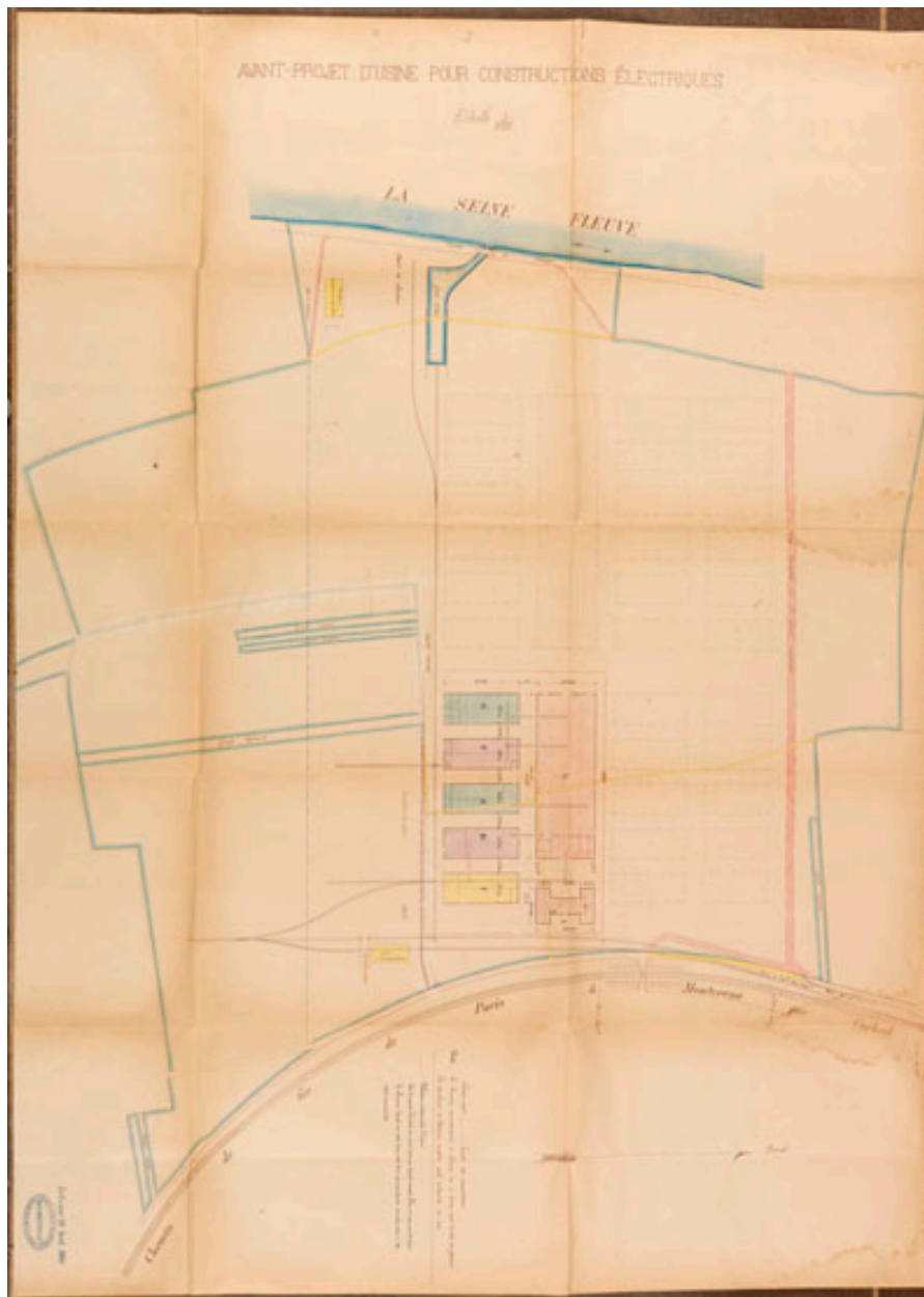
Avant projet d'usine pour construction électrique. Plan Echelle 1/1000e.
