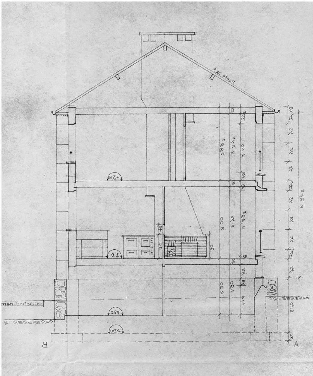
Coupe d'un pavillon.
