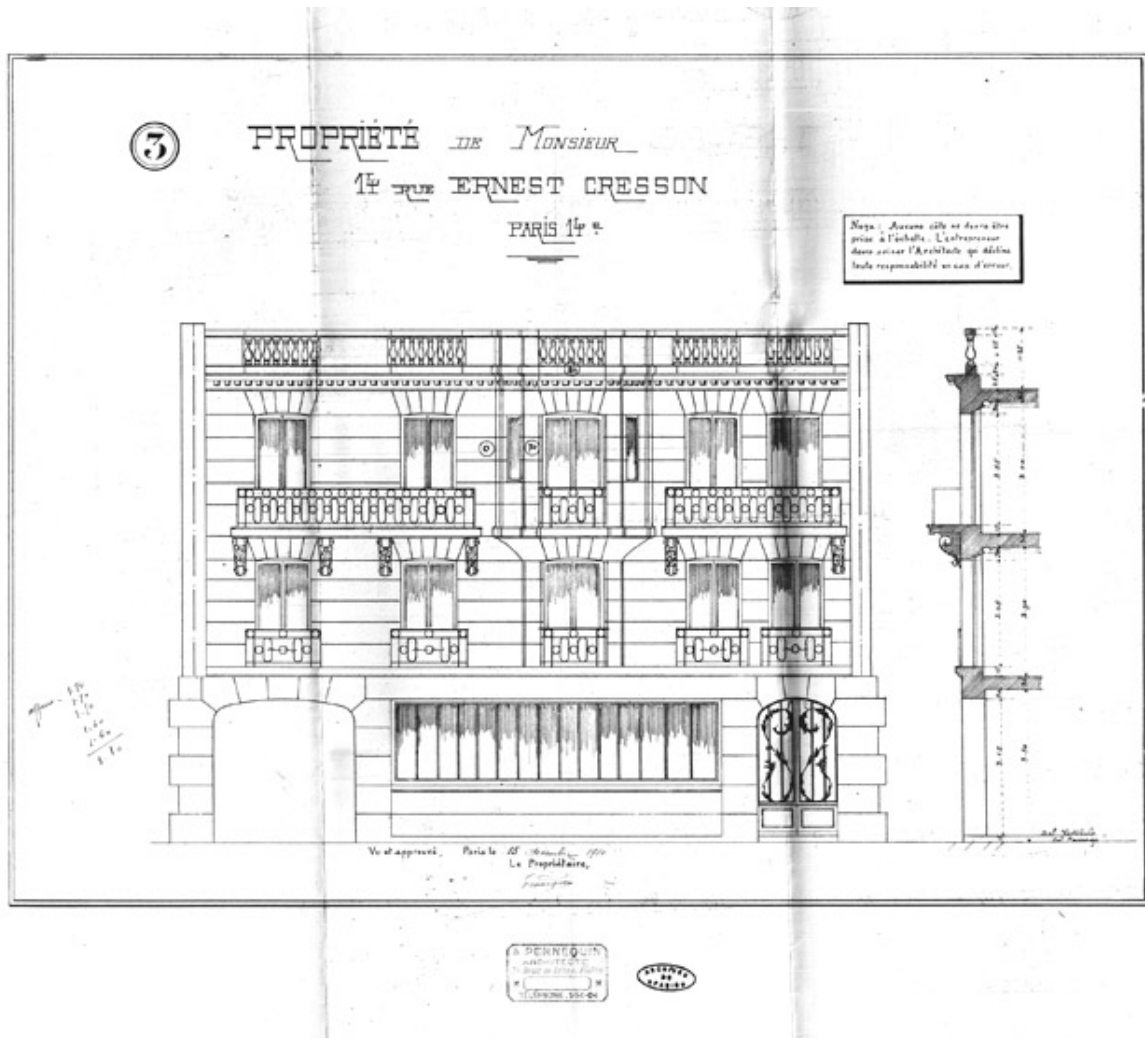
Facade, élévation dressée par A.Pennequin, architecte.-Pla, 1910. (Archives de Paris. VO11 1131).
