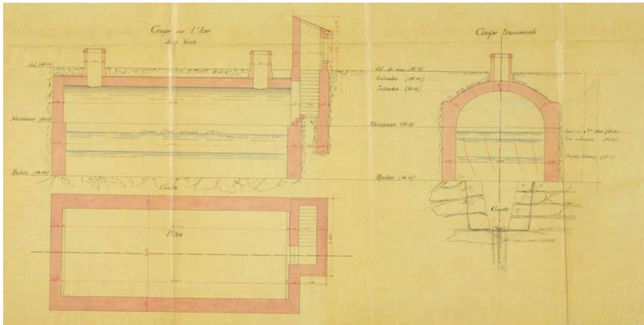
Plan et coupes de la prise d'eau établie à Valvins, en 1855, pour l'alimentation des bornes fontaines de Fontainebleau. (AD Seine-et-Marne, 3353W1169 )
